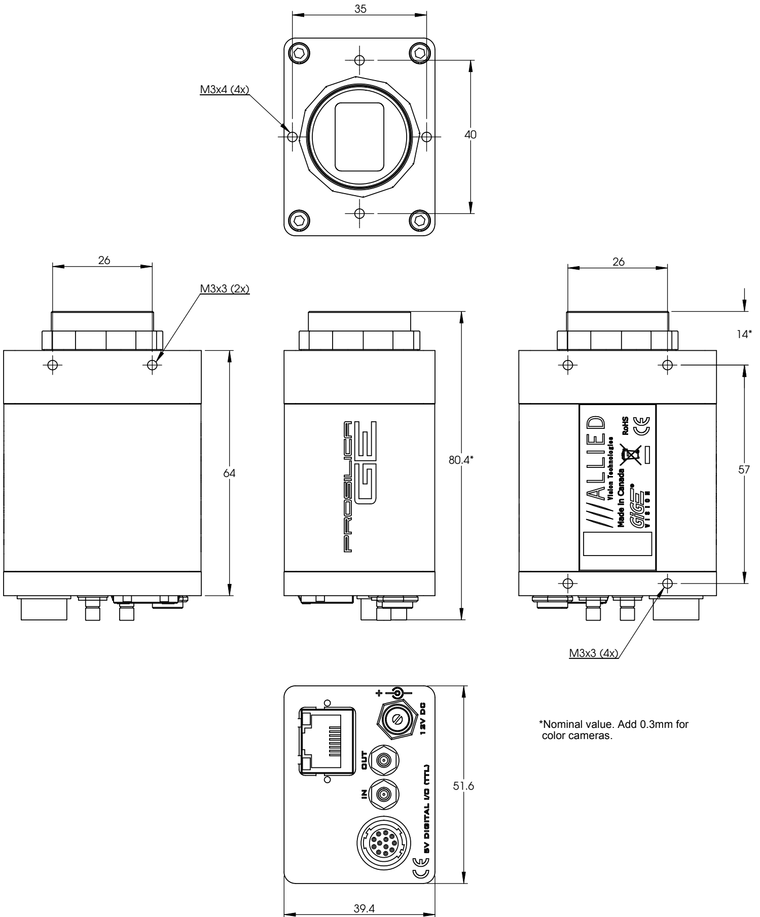
Prosilica GE1650
